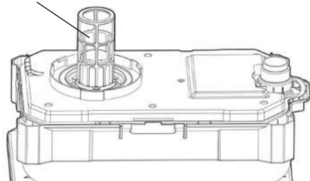
Корпус поплавка
